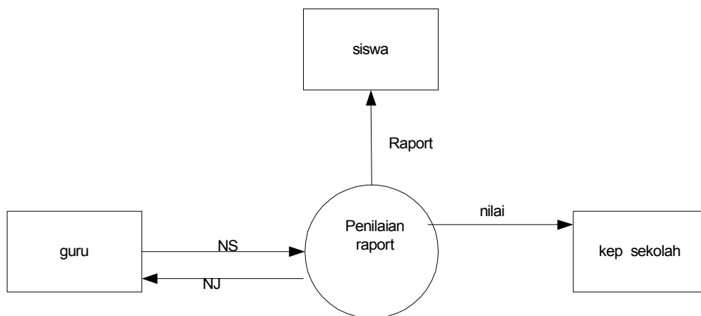
Gambar 4.1 Diagram Konteks
